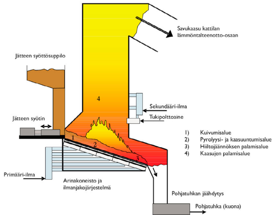
Kuva 5-2 Arinapoltton periaatekaavio
