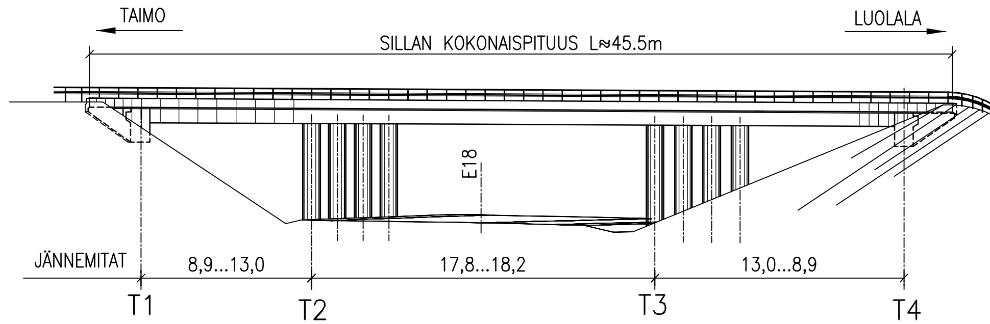
SIVUKUVA 1:200
