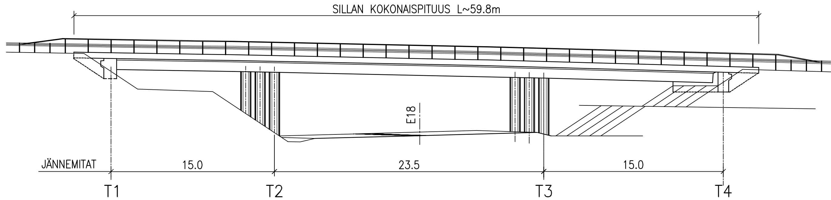
TASOKUVA 1:200
