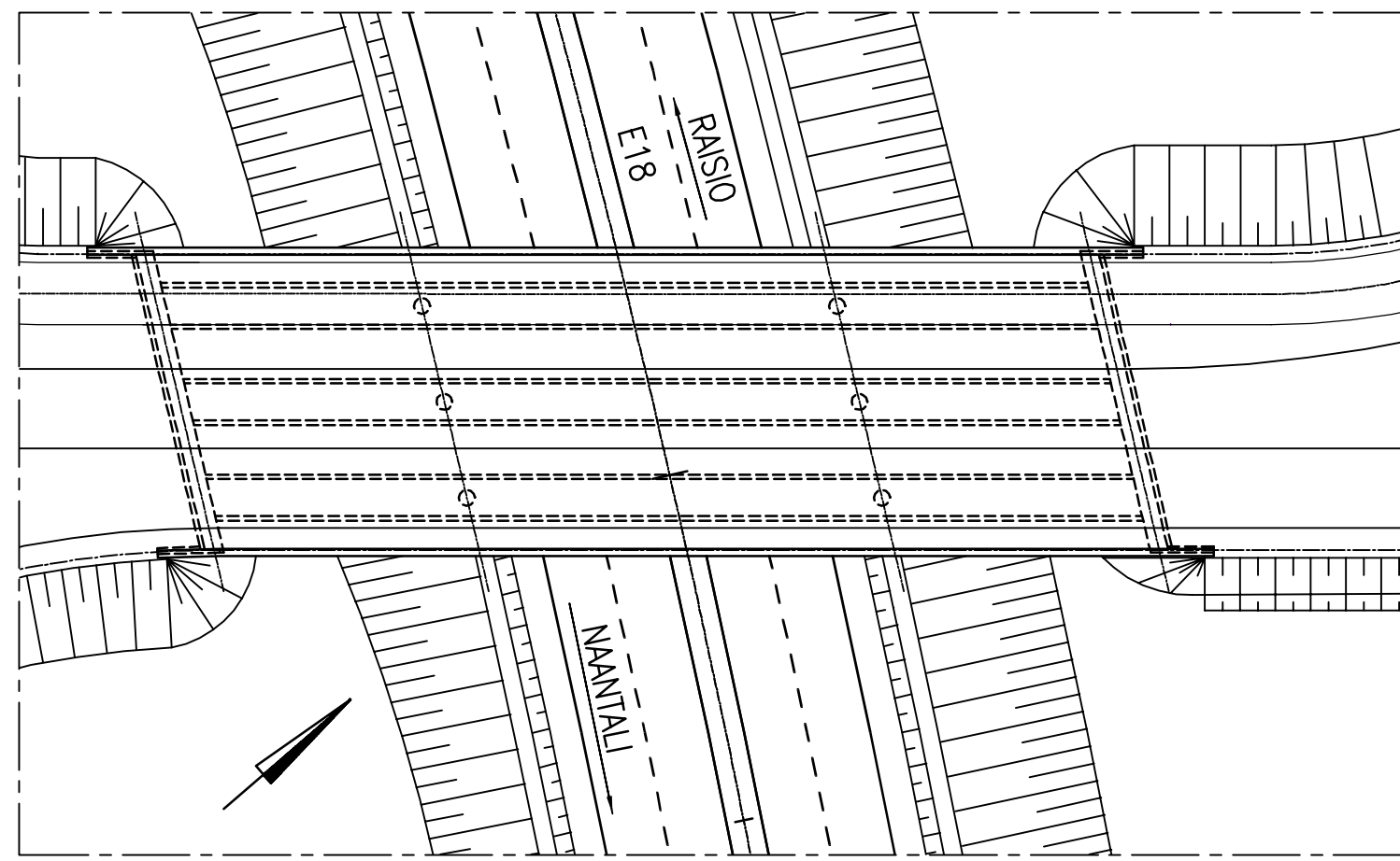
TASOKUVA 1:500
