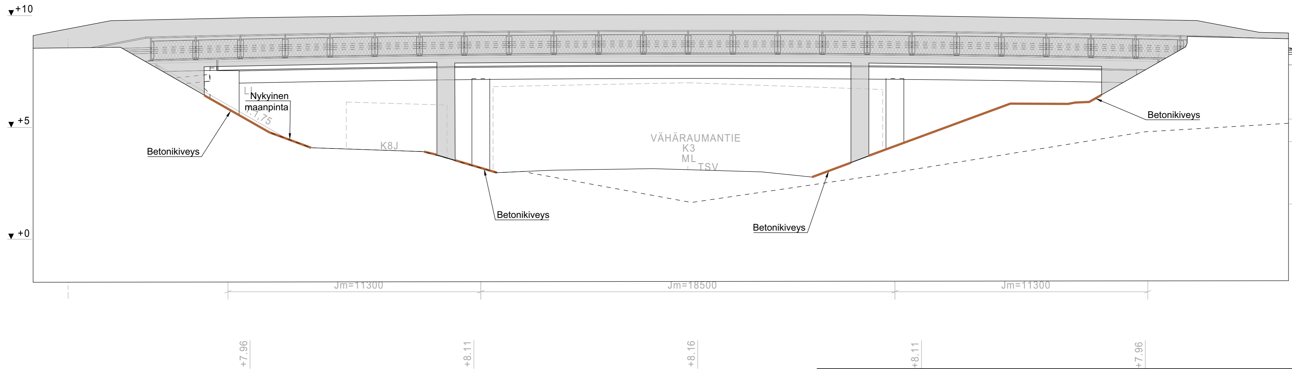
S2 A-A 1:100
